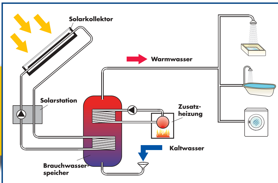
Funktionsprinzip einer Solarthermischen Anlage
