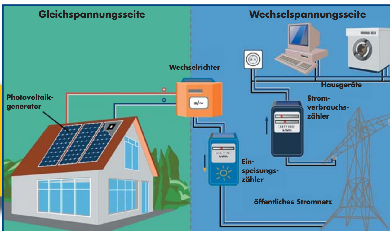
Funktionsprinzip einer Photovoltaik-Anlage
