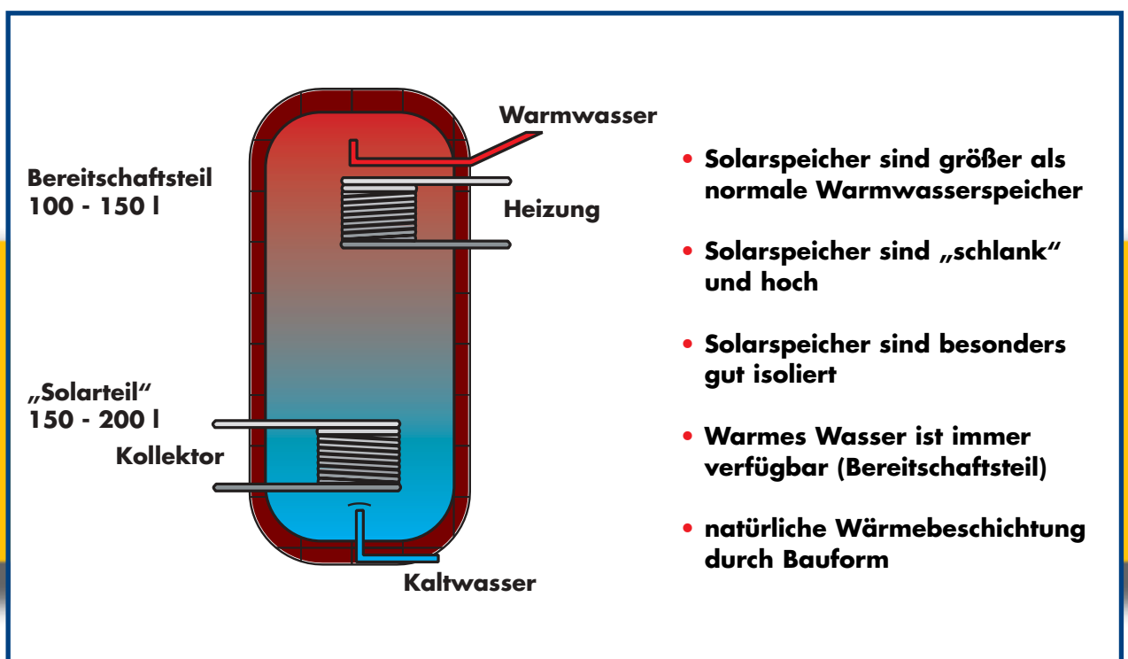
Der Brauchwasserspeicher
